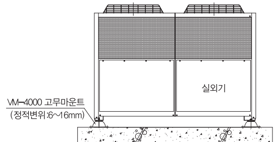
E.H.P 실외기 방진 상세도
