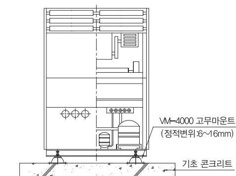
팩케이지 에어컨 방진 상세도
